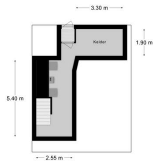
Souterrain
